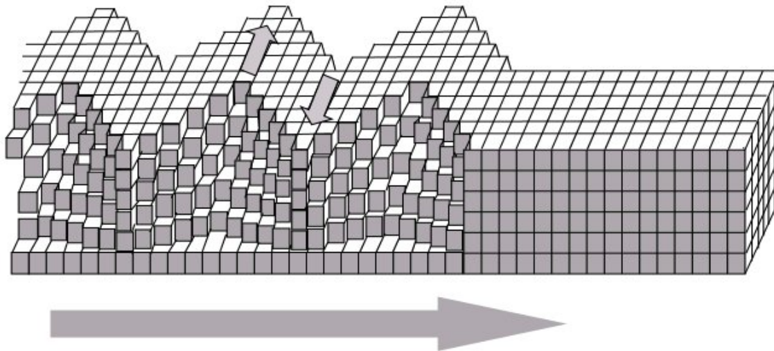
Love Wave
