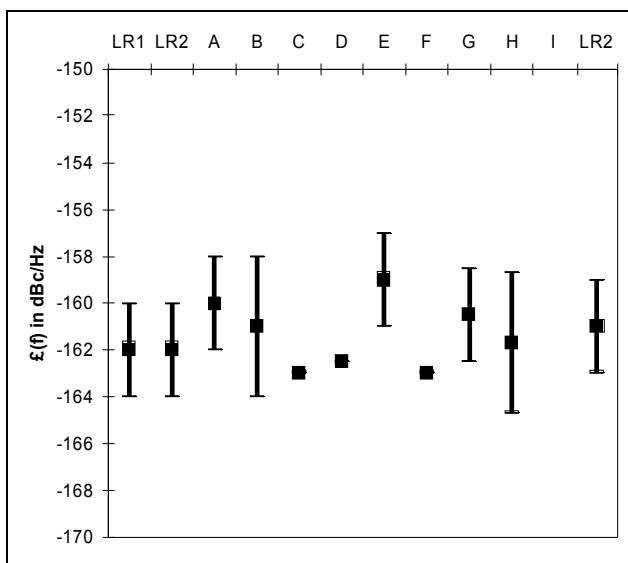
Mesures à 100 kHz pour une porteuse à 100 MHz. Incertitudes sont données à 2\sigma
