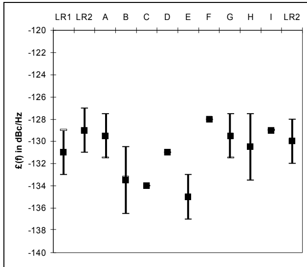
Mesures à 100 Hz pour une porteuse à 100 MHz. Incertitudes sont données à 2\sigma
