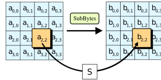
SubBytes
