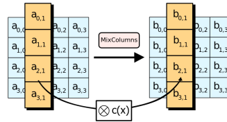
MixColumns
